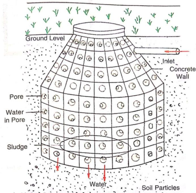
Fig.6.1: Cesspool
